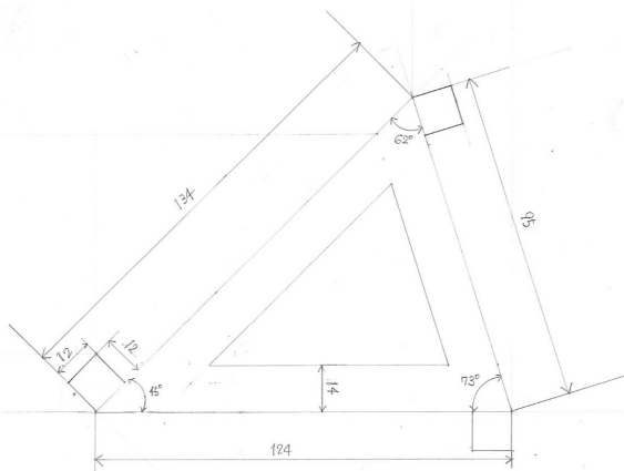
スマホスタンド図面 現寸
